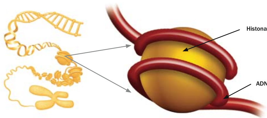
Histonas. Cuando las señales de la célula ocasionan que las histonas se compacten, las moléculas que leen el código no pueden tener acceso al ADN, con lo cual se “apaga” el gen. Cuando las señales de la célula permiten que las histonas se separen entre sí, las moléculas pueden entonces leer el ADN y el gen está “activo”.
